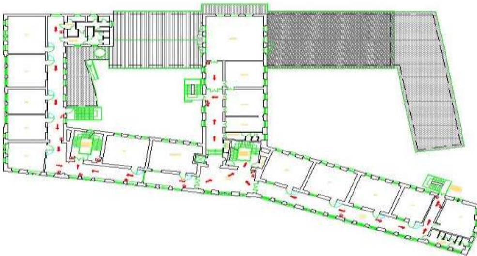
PIANO PRIMO
